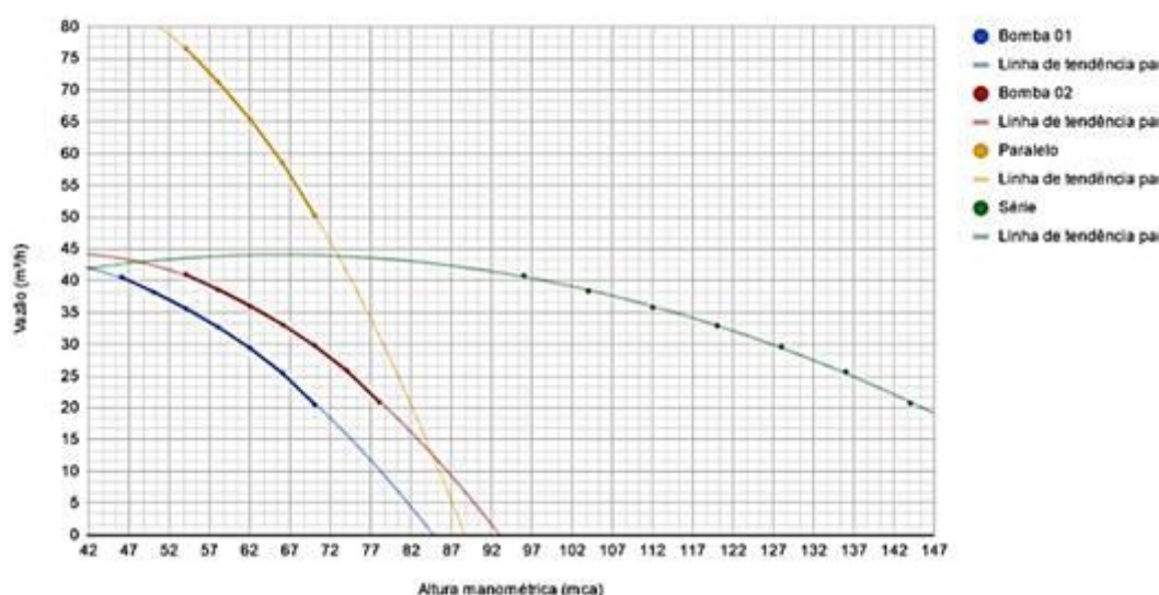
Associação de bombas
