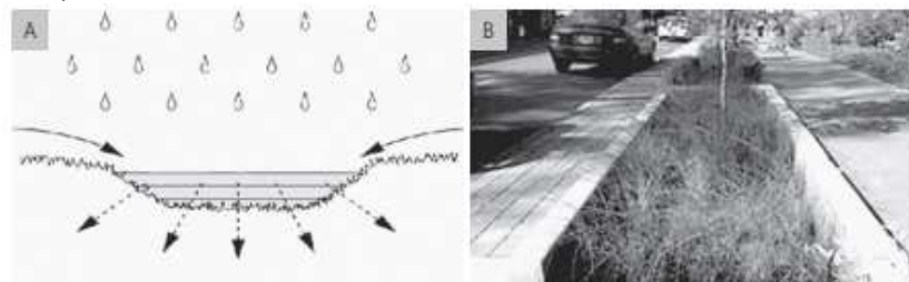
Figura 1.12 Bacia de infiltração.
