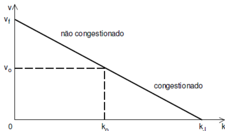
Figura 3.4 Representação gráfica do modelo linear de velocidade-concentração
